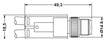
Y-kontakt M 12 x 1
