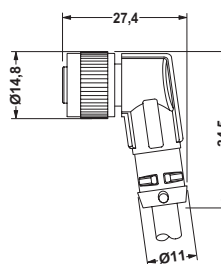
Hona M 12 x 1, vinklat utförande
