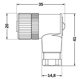
Hona M 12 x 1, vinklat utförande
