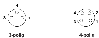
Polbild M 8-kontakt (hona)
