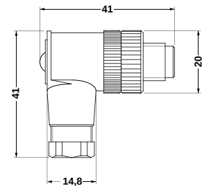
Hane M 12 x 1, vinklat utförande
