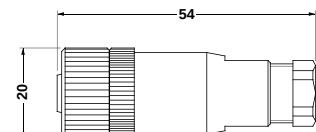
Hona M 12 x 1, rakt utförande
