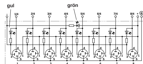
Plint-konfiguration: SACB-QUICKON SC (för pnp-sensorer / aktorer)
