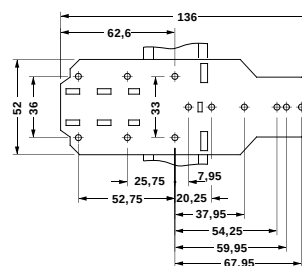
montageplatta UTA 136
