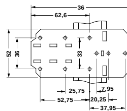
montageplatta UTA 107
